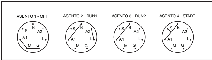
PÄÄKYTKINTEN ASENNOT
