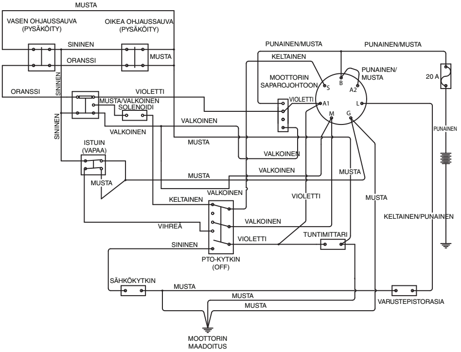
PÄÄKYTKINTEN ASENNOT
