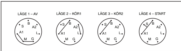
NYCKELBRYTARE, LÅGEN
